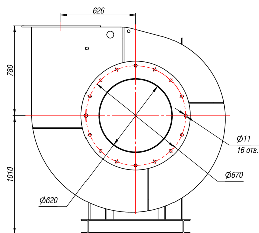
Выходной фланец
