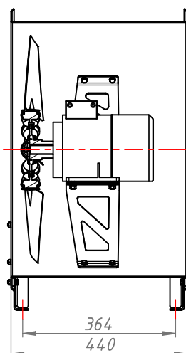
71/80 габарит ЭД
