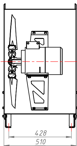
80/90/100 габарит ЭД
