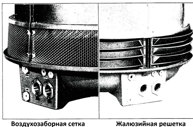
Рисунок 1.4.7. Воздухозаборное устройство
