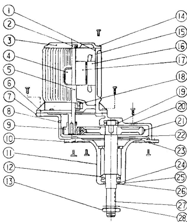
Рисунок 2.5. Конструкция редукторного электродвигателя
