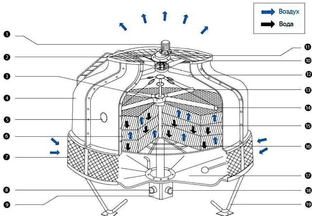
Рисунок 1.4.1. Конструкция градирни
