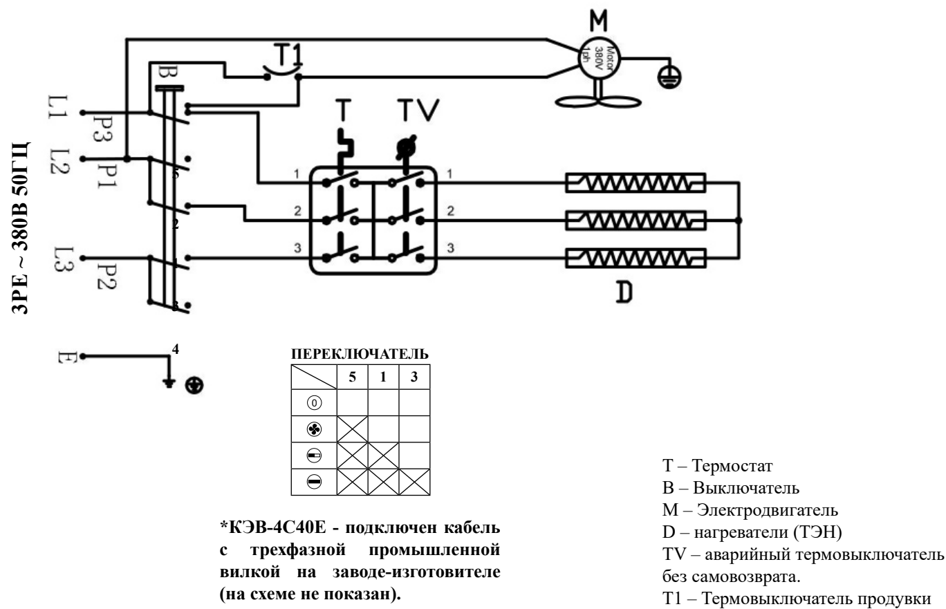
Рисунок 10. Электрическая схема тепловентиляторов КЭВ-4С40Е*, КЭВ-6С40Е и КЭВ-9С40Е
