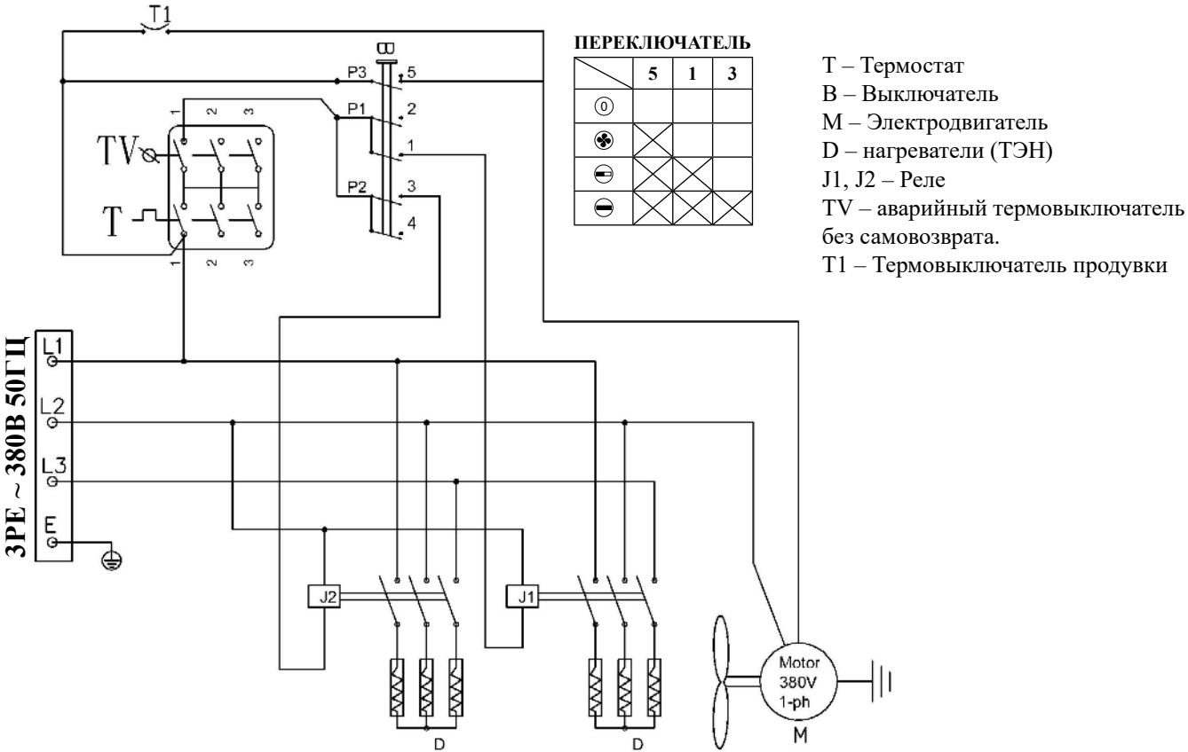
Рисунок 12. Электрическая схема тепловентилятора КЭВ-18С40Е
