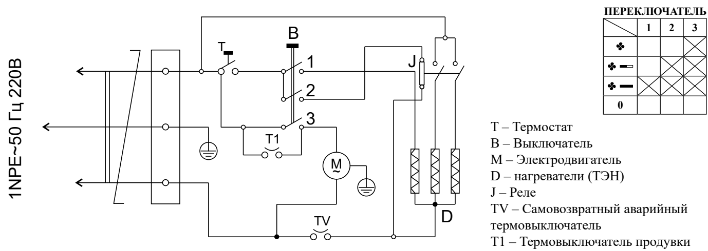
Рисунок 8. Электрическая схема тепловентилятора КЭВ-4С41Е
