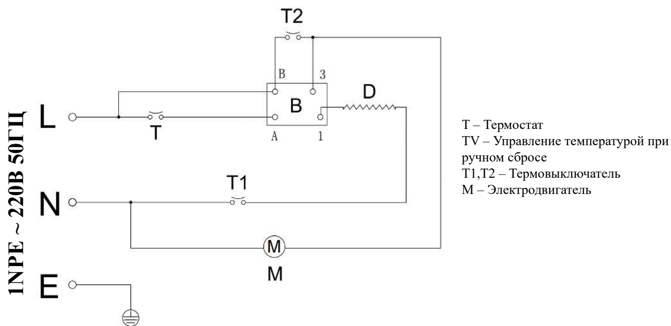
Рисунок 3. Электрическая схема тепловентилятора КЭВ-2С31Е, КЭВ-3С31Е
