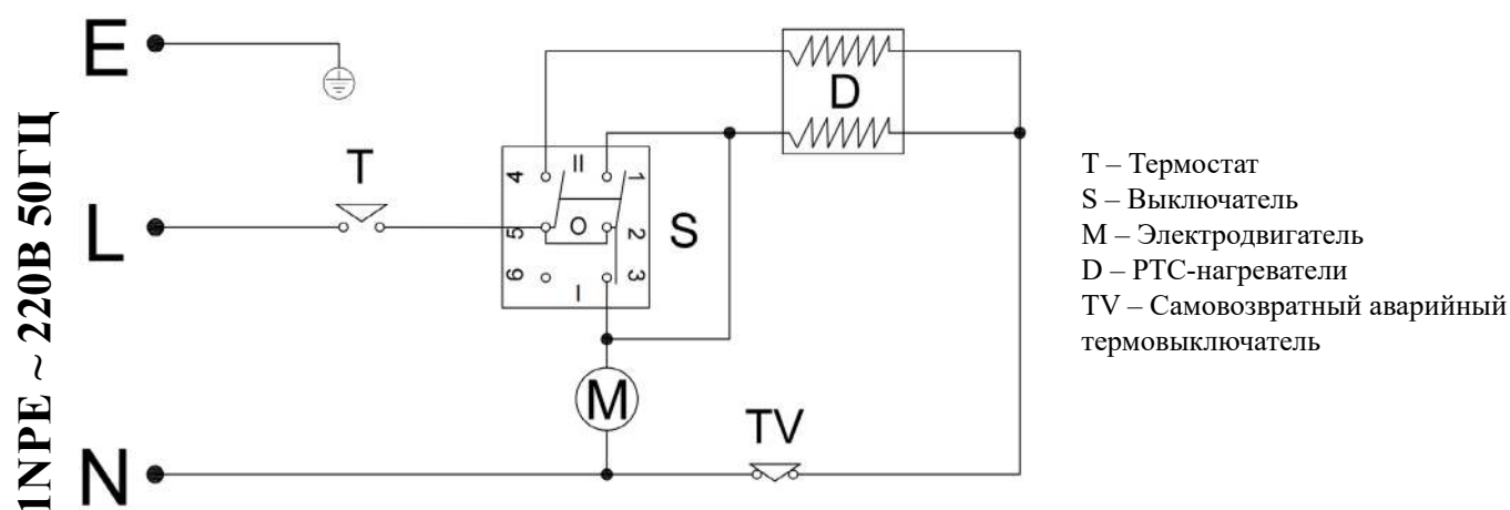
Рисунок 3. Электрическая схема тепловентилятора КЭВ-2С31Е, КЭВ-3С31Е
