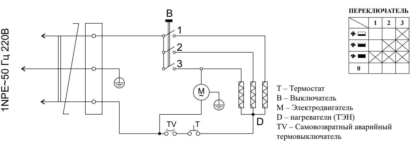
Рисунок 5. Электрическая схема тепловентилятора КЭВ-2С41Е
