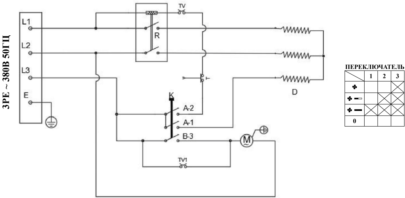
Рисунок 7. Электрическая схема тепловентилятора КЭВ-5С31Е
