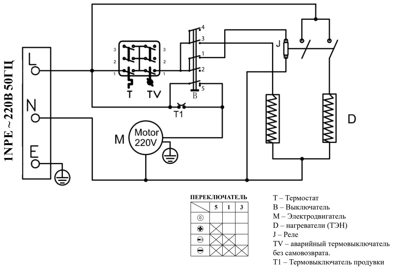
Рисунок 9. Электрическая схема тепловентилятора КЭВ-6С41Е
