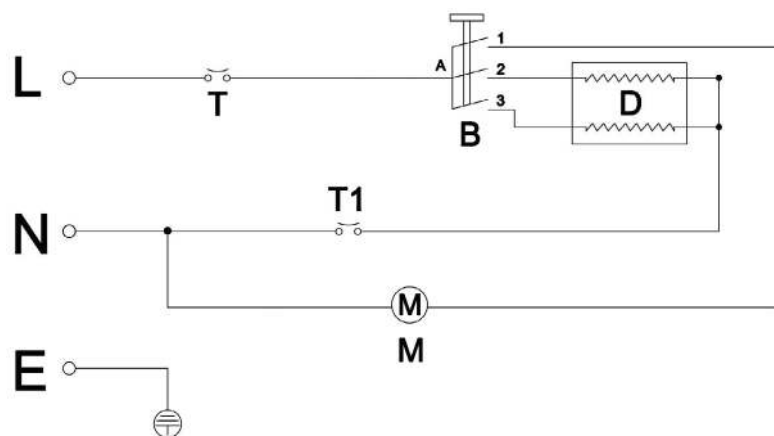
Рисунок 4. Электрическая схема тепловентилятора КЭВ-2С61Е
