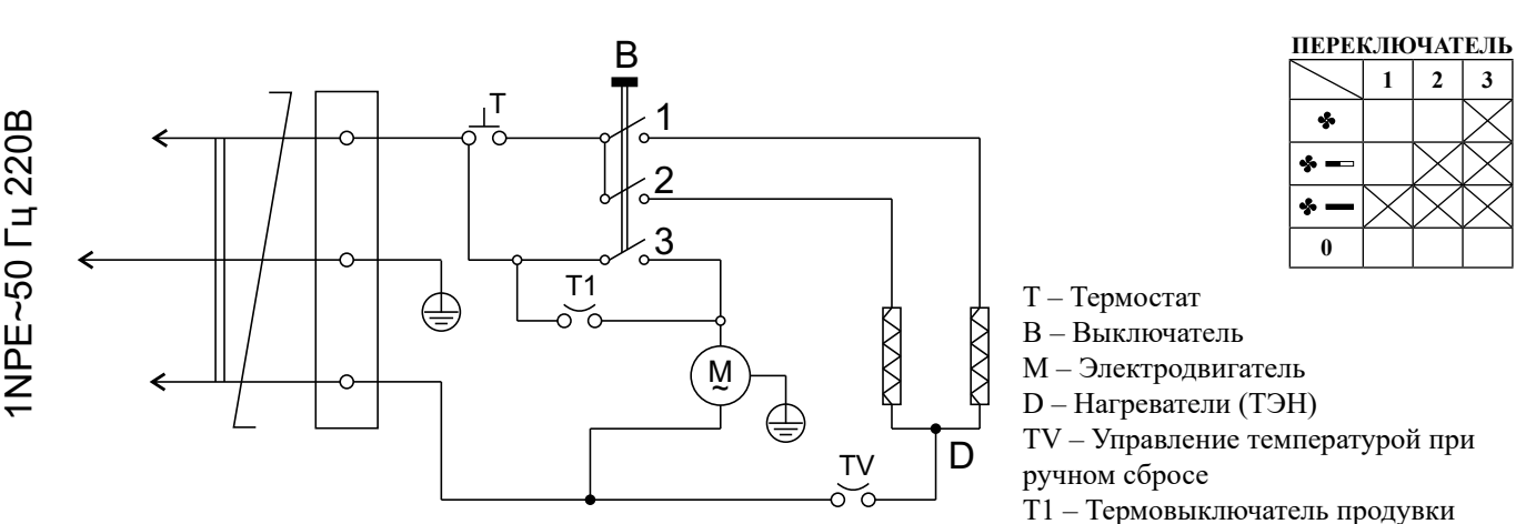
Рисунок 6. Электрическая схема тепловентилятора КЭВ-3С41Е
