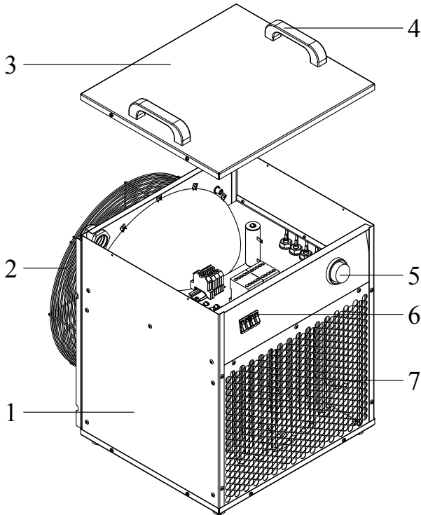
Рисунок 1. Тепловентилятор
