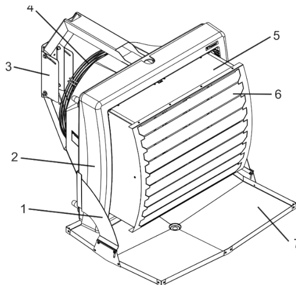
Рисунок 1 - Фанкойл
