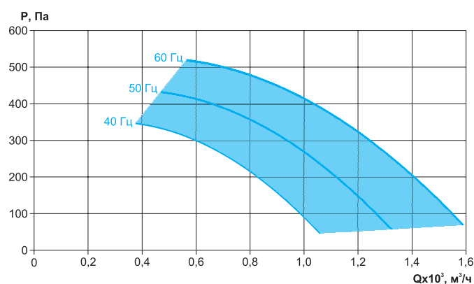
ВРС-К-50-30/22-РК635-0,18/3000/220-380
