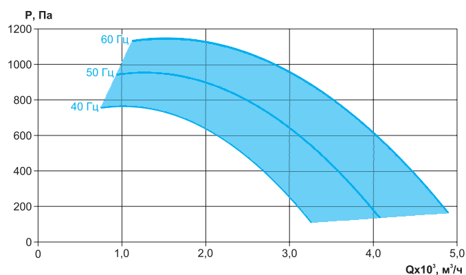
ВРС-К-60-35/31-РК635-1,5/3000/220-380
