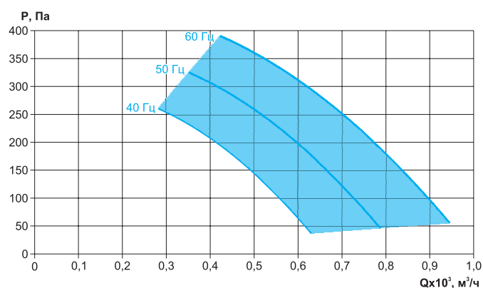
ВРС-К-40-20/18-РК635-0,18/3000/220-380
