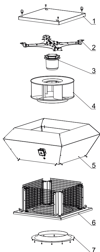
Рисунок 1.1 – Состав вентилятора ВКРФ-М с рабочим колесом ГН
