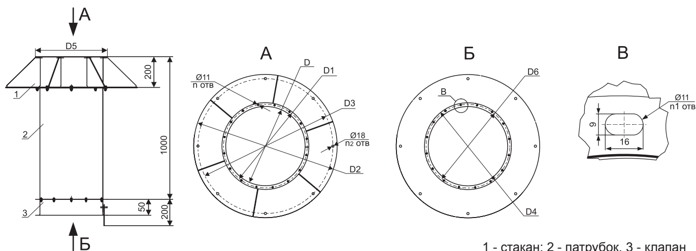
1 - стакан; 2 - патрубок, 3 - клапан
