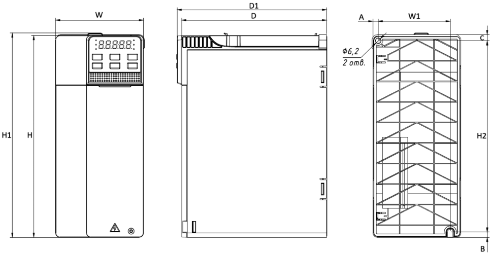
Рисунок 3.6-3 – Чертеж преобразователя частоты типоразмера С3
