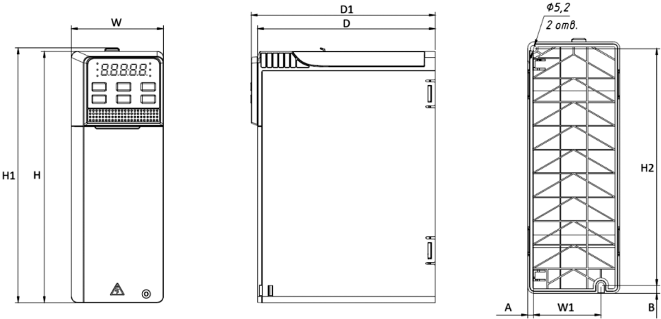
Рисунок 3.6-2 – Чертеж преобразователя частоты типоразмера C2
