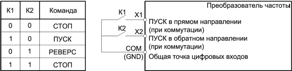
Рисунок 10.9-5 – Двухпроводная схема управления 1
