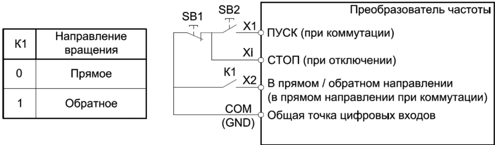
Рисунок 10.9-7 – Трёхпроводная схема управления 1
