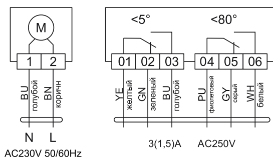
Рисунок 6.3 – Схемы подключения приводов BLF
