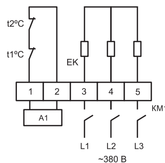
Схема подключения ЭНК-2 на 380В
