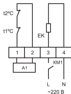
Схема подключения ЭНК-1 на 220В
