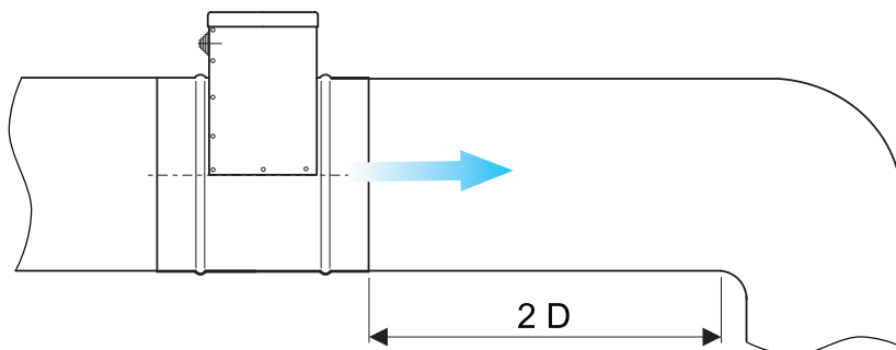
Рисунок 5.1 – Минимальное расстояние до изгиба канала
