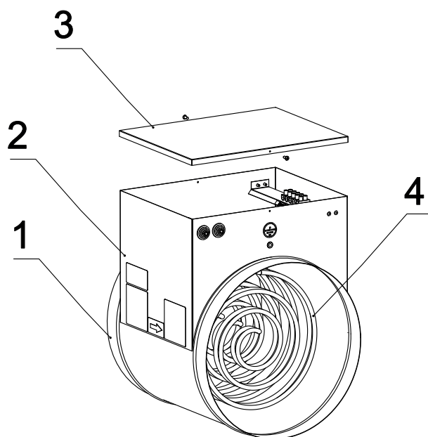
Рисунок 1.1 – Состав электронагревателя ЭНК
