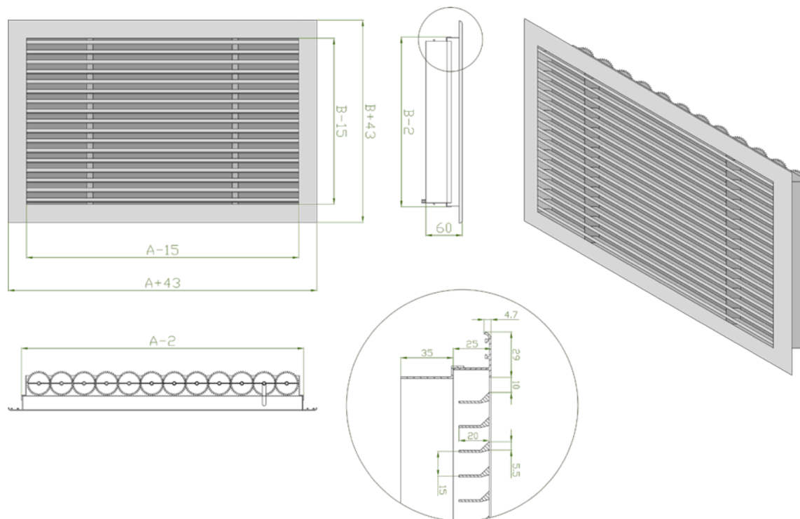
Габаритно-посадочные размеры регулируемой решетки ННРБ-Y AxB размеры строительного проема.
