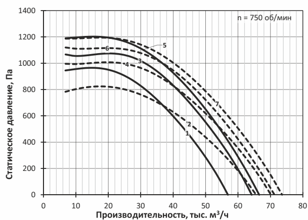
mrc PASSAT-V-K-12,5
