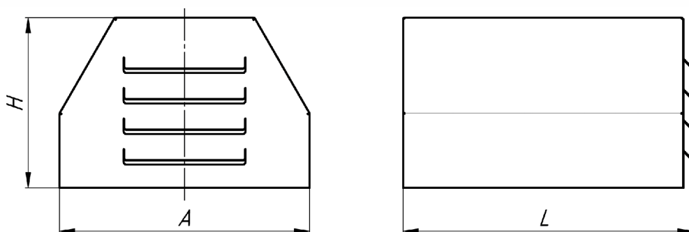
Габаритно-присоединительные размеры
