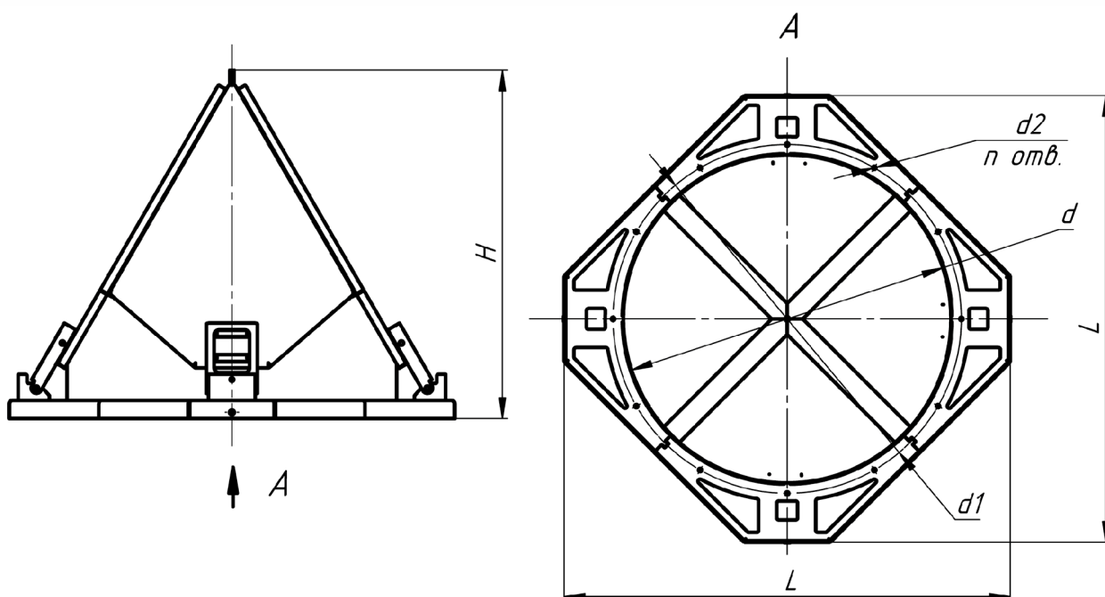
Габаритно-присоединительные размеры
