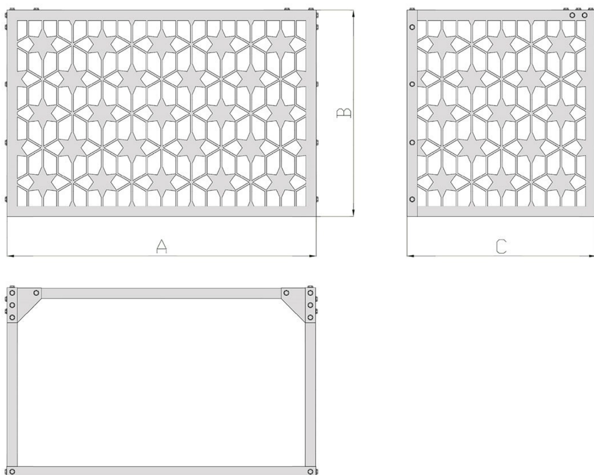
Панель для кондиционера AIRS ПДНБ-Декор
