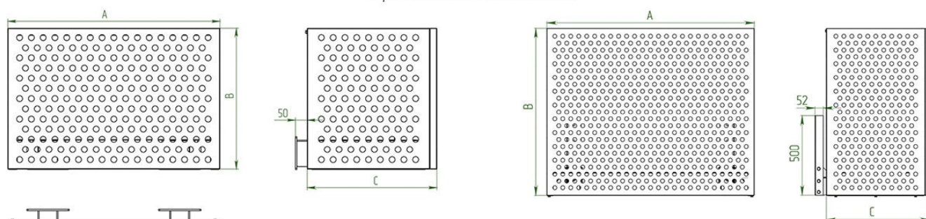
Корзина AIRS LiteBox LB-2-P-Lv-KФ
