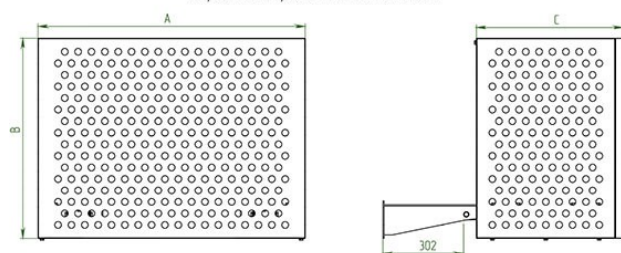
Корзина с кронштейном AKFU-P
