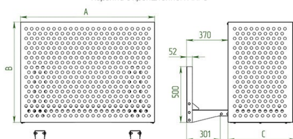
Корзина с кронштейном AKFU
