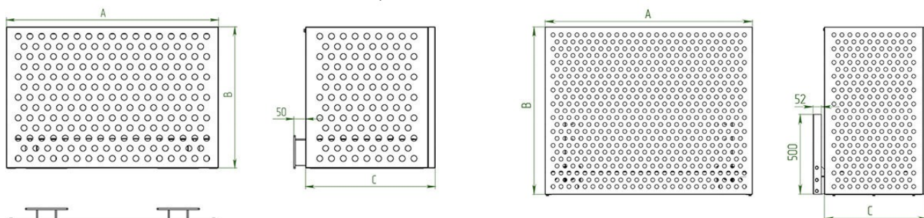
Корзина AIRS LiteBox LB-1-P-Qd-KФ
