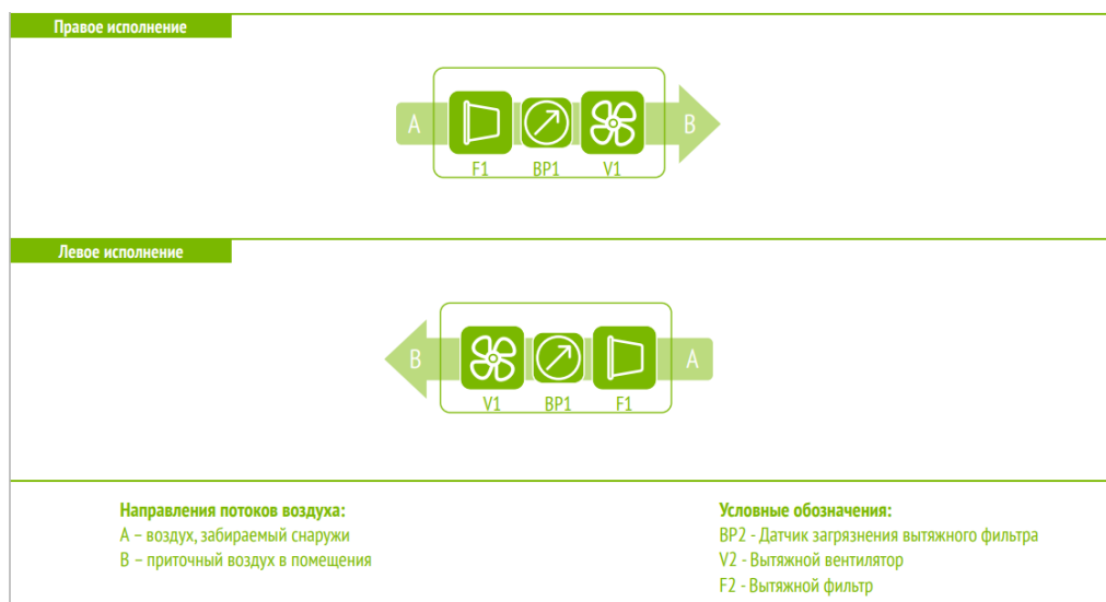
Рисунок 12.1. Функциональная схема установок ОТД–Е
