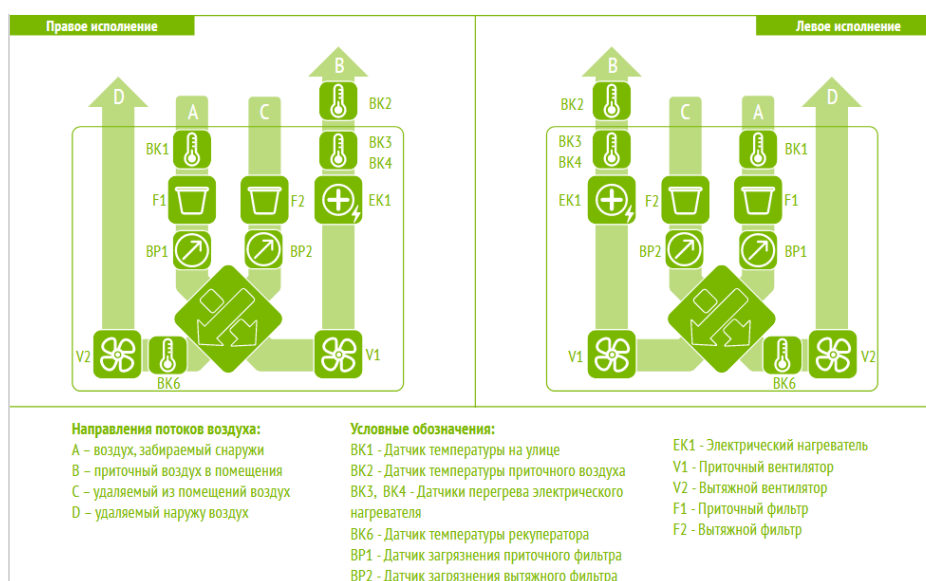
Рисунок 5. Функциональная схема установок ОТД-P-...-V-E
