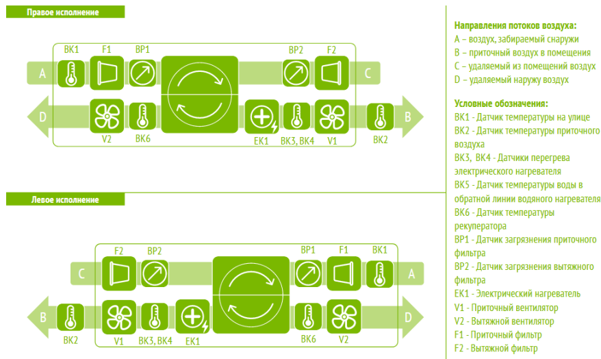
Рисунок 7. Функциональная схема установок ОТД–R-1000_1500_2000_3000-U,1300-F
