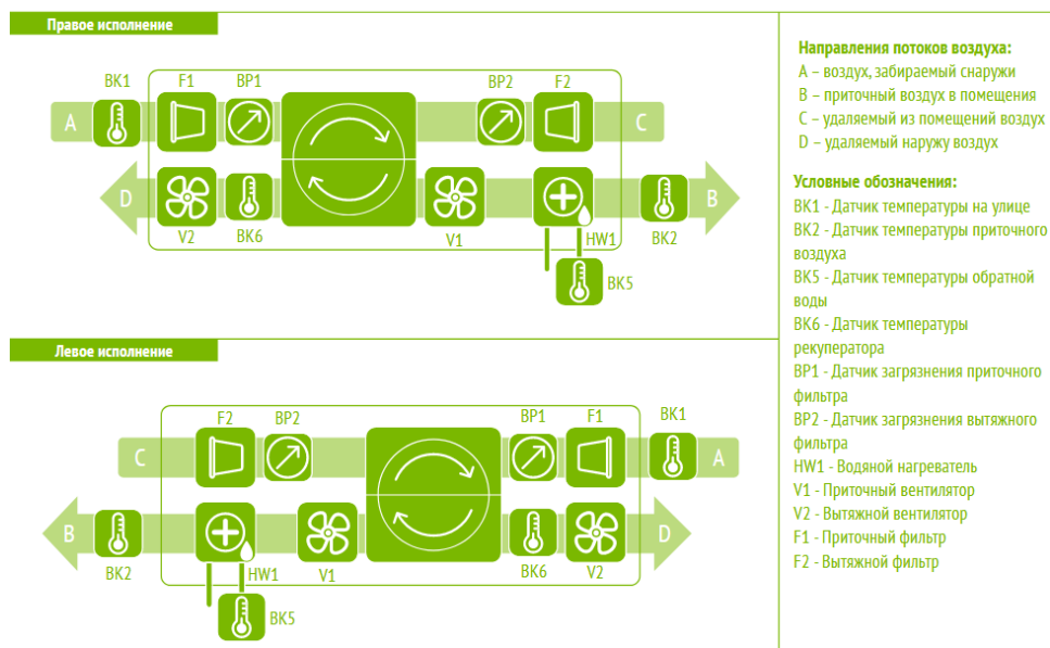
Рисунок 9. Функциональная схема установок ОТД–R-1000_1500_2000_3000-U
