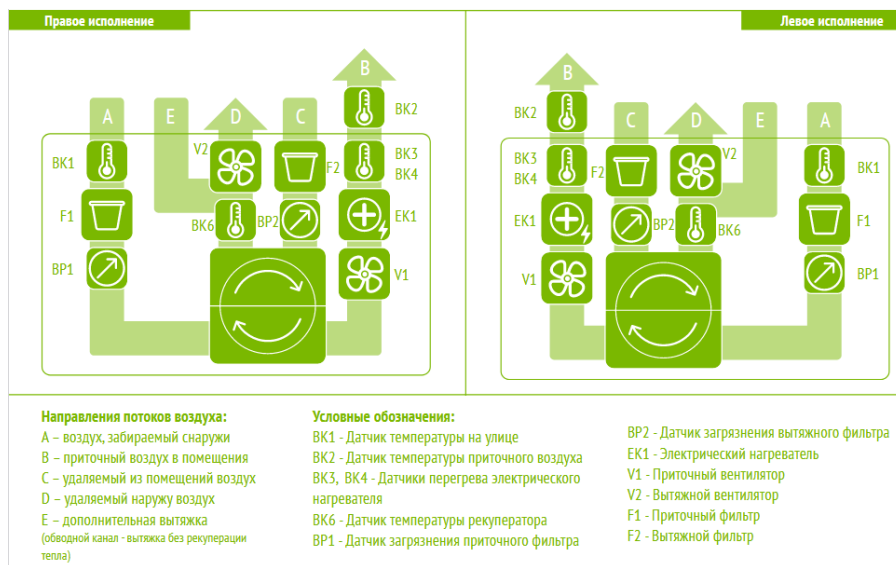
Рисунок 8. Функциональная схема установок ОТД–R-300_400_500_700-V
