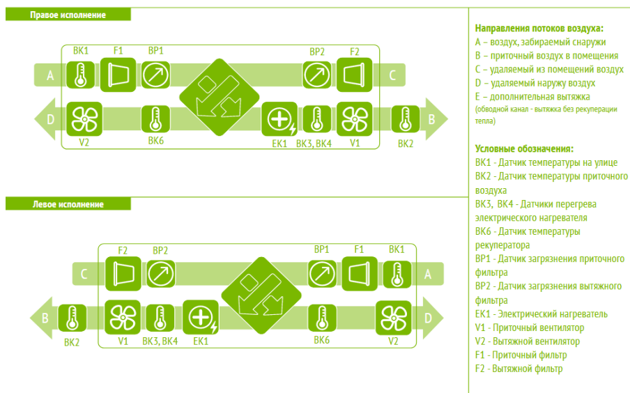
Рисунок 1. Функциональная схема установок ОТД – Р-600-Ф
