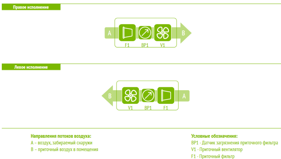
Рисунок 12. Функциональная схема установок ОТД-S-X
