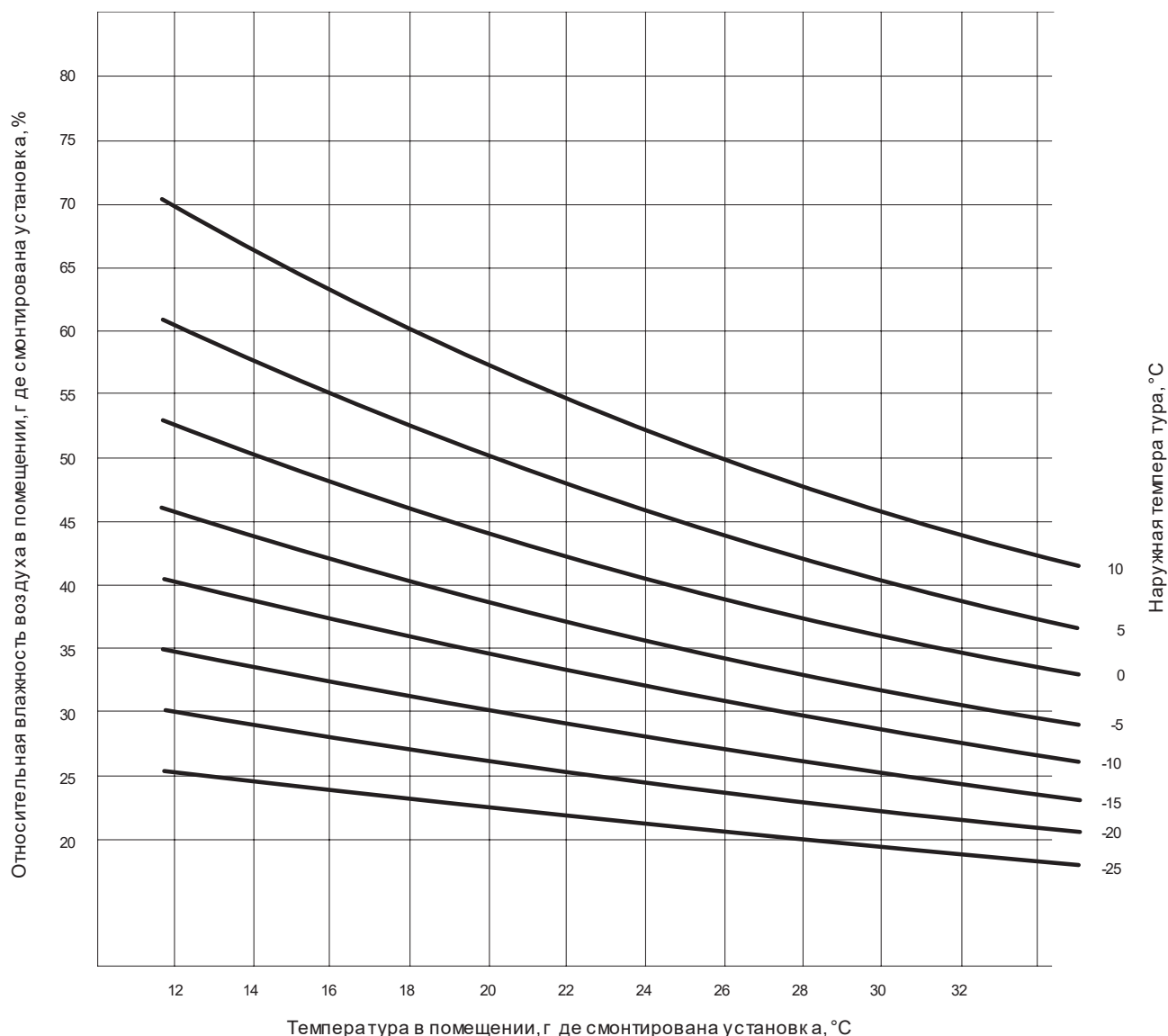
Рисунок 13 – График образования конденсата
