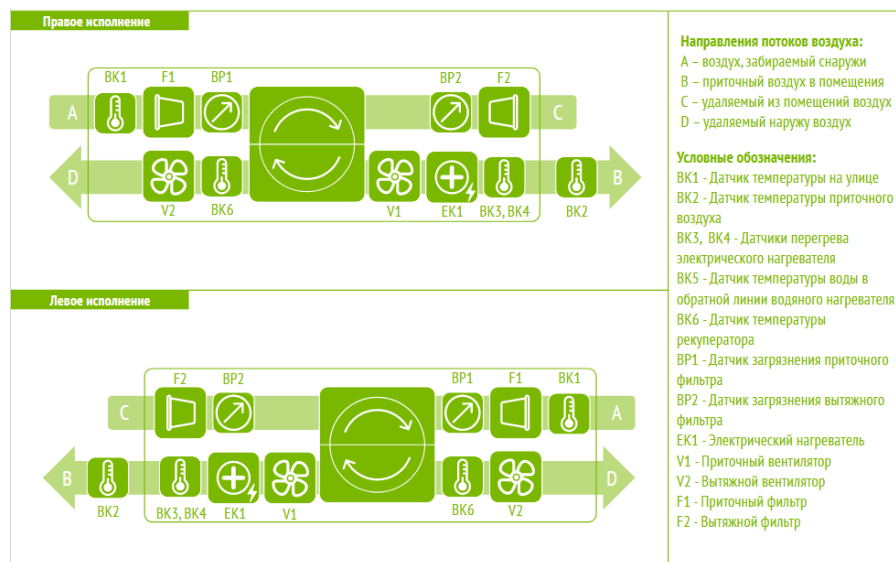
Рисунок 4. Функциональная схема установок ОТД-R-500_700-Н
