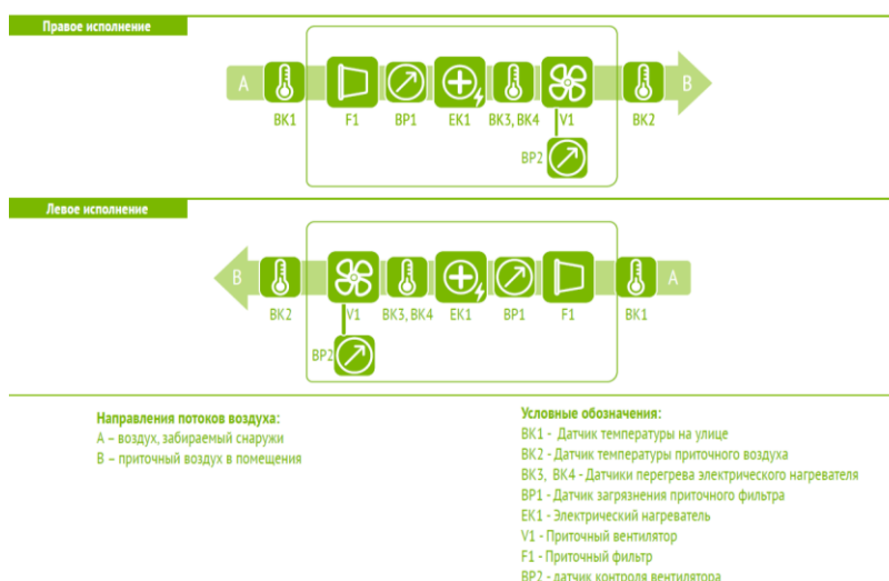
Рисунок 5. Функциональная схема установок ОТД-P-...-V-E
