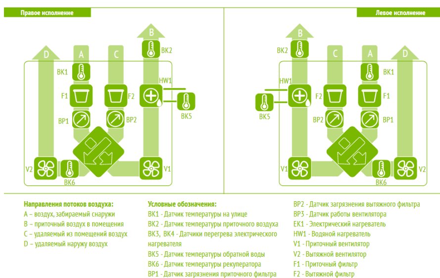
Рисунок 2. Функциональная схема установок ОТД – Р-...-V-W
