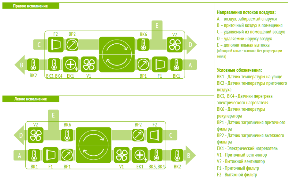
Рисунок 10. Функциональная схема установок ОТД-R-250-F
