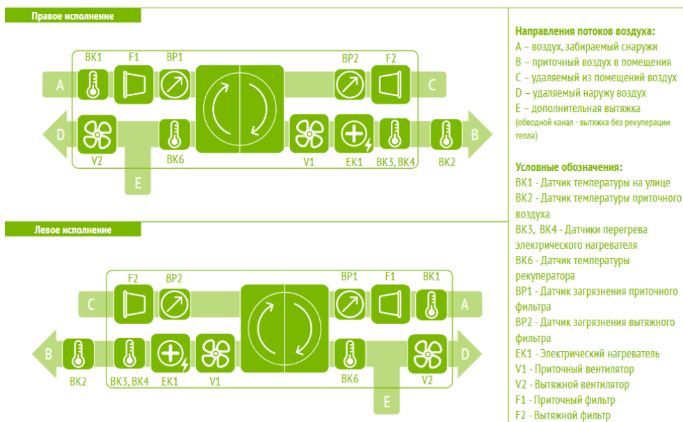
Рисунок 11. Функциональная схема установок ОТД-R-400_700-F
