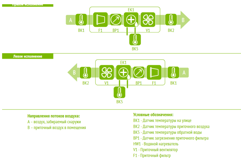
Рисунок 3. Функциональная схема установок ОТД-S-W
