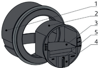
Клапаны постоянного расхода воздуха KOMFIX-P
