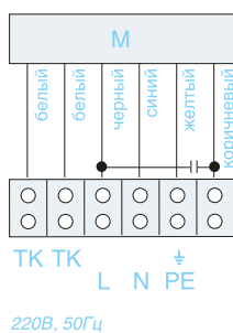
1-фазный двигатель
