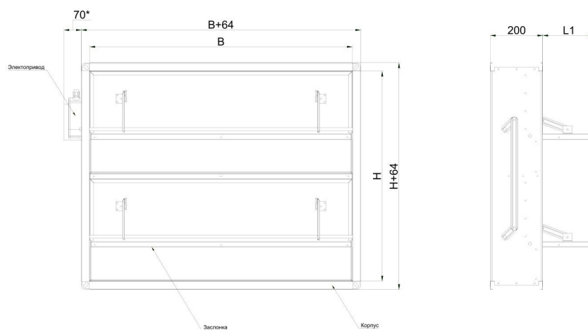
Чертёж клапана EI 120
