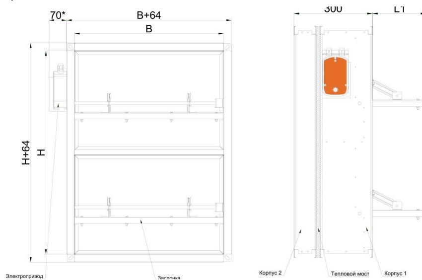
Чертёж клапана EI 120
