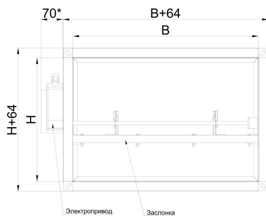
Чертёж клапана EI 120
