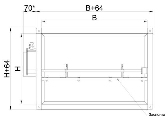
Чертёж клапана EI 120
