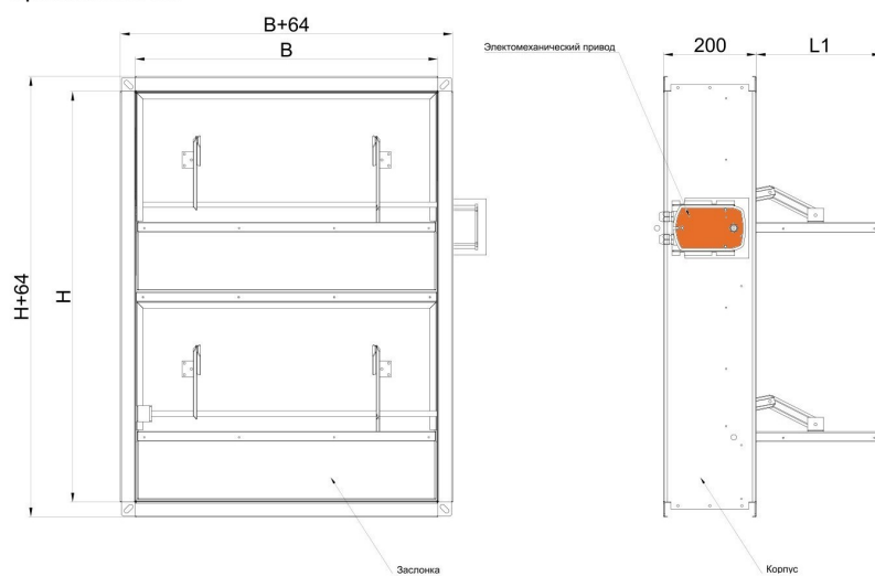
Чертёж клапана EI 120
