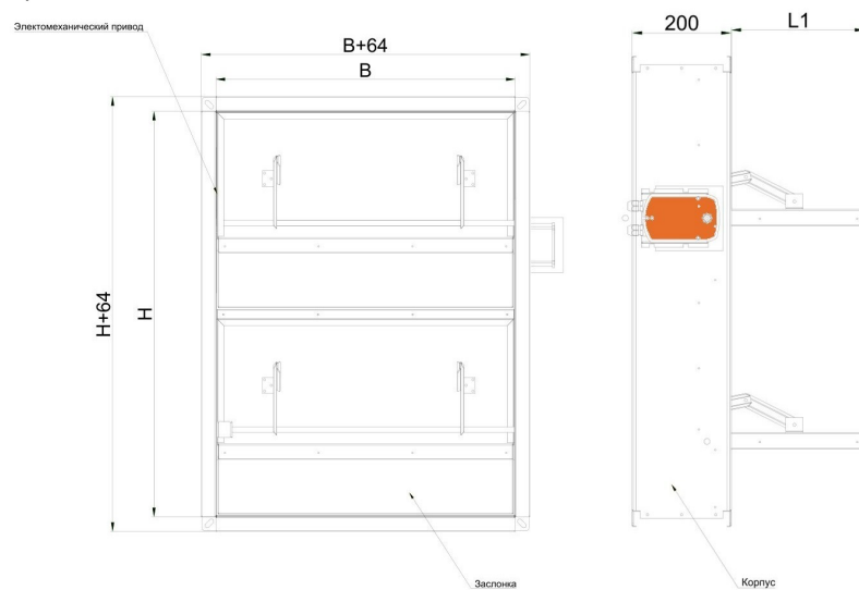
Чертёж клапана EI 120
