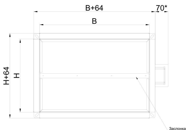
Чертёж клапана EI 120
