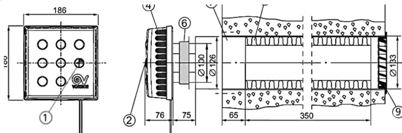
Схема клапана КИВ Квадро. Все размеры приведены в мм.
