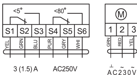
Схемы электрических подключений
