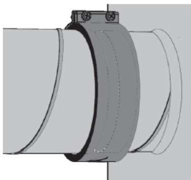
Пример использования быстросъемного хомута
