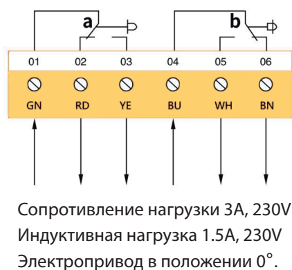
Вспомогательный переключатель
