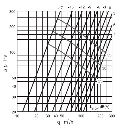
Открытие диффузора DVS 125 в мм
