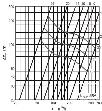
Открытие диффузора DVS 200 в мм
