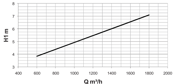
DFAZ-2 315mm Вертикальный поток \Delta T= 10\text{ C}
