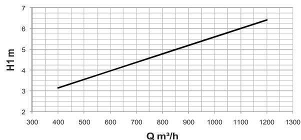
DFAZ-2 250mm Вертикальный поток \Delta T= 10\text{ C}
