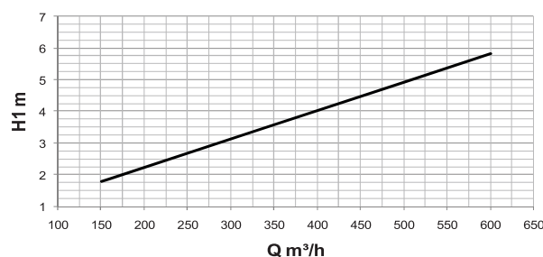
DFAZ-2 160mm Вертикальный поток \Delta T= 10\text{ C}
