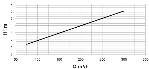
DFAZ-2 100mm Вертикальный поток \Delta T= 10\text{ C}
