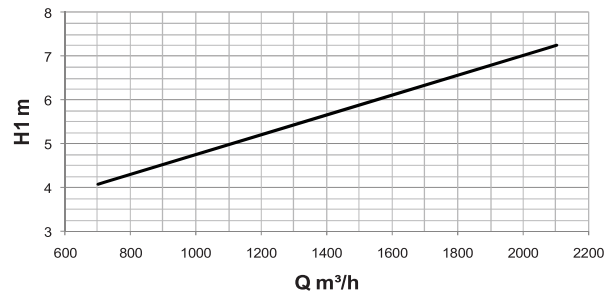
DFAZ-2 350mm Вертикальный поток \Delta T= 10\text{ C}
