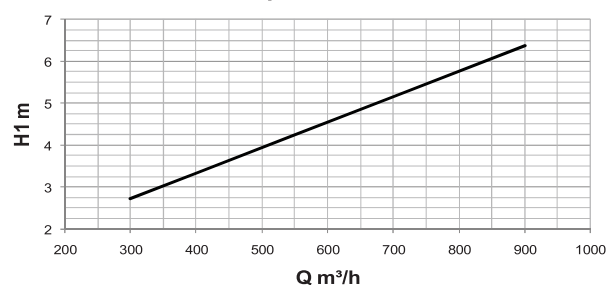
DFAZ-2 200mm Вертикальный поток \Delta T= 10\text{ C}
