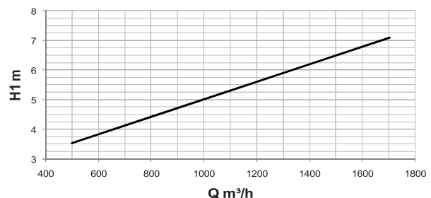
DFAZ-2 300mm Вертикальный поток \Delta T= 10\text{ C}
