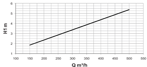
DFAZ-2 150mm Вертикальный поток \Delta T= 10\text{ C}
