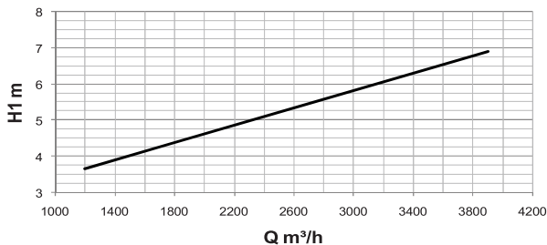
DFAZ-2 500mm Вертикальный поток \Delta T = 10\text{ C}
