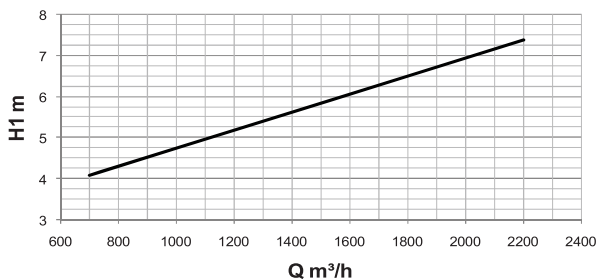
DFAZ-2 355mm Вертикальный поток \Delta T = 10\text{ C}
