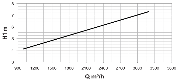
DFAZ-2 450mm Вертикальный поток \Delta T = 10\text{ C}
