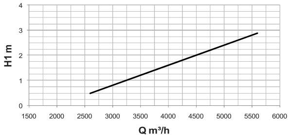
DFAZ-2 630mm Вертикальный поток \Delta T = 10\text{ C}
