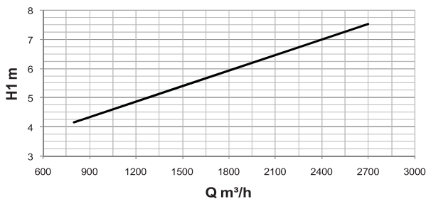
DFAZ-2 400mm Вертикальный поток \Delta T = 10\text{ C}
