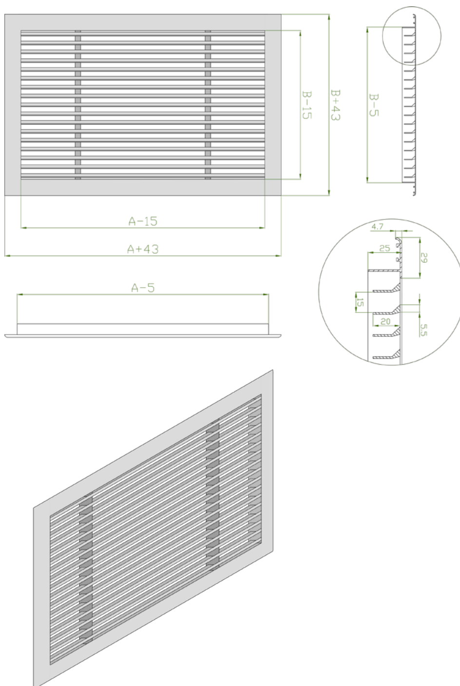
Габаритно-посадочные размеры регулируемой решетки ННР-У A \times B размеры строительного проема.
