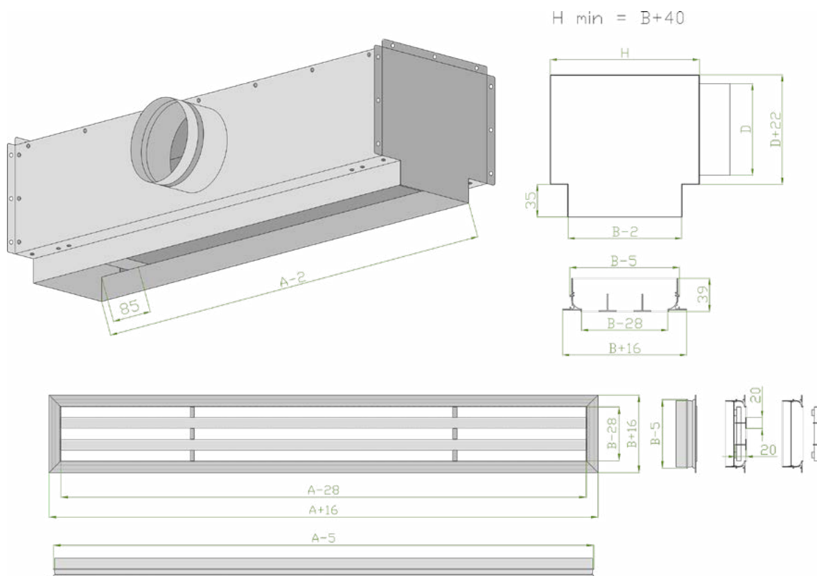
F1 Одиночная секция с фланцами
