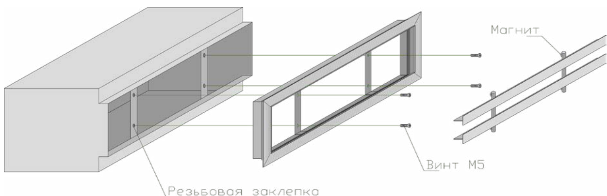
Монтаж щелевой решетки G-Line-TS
