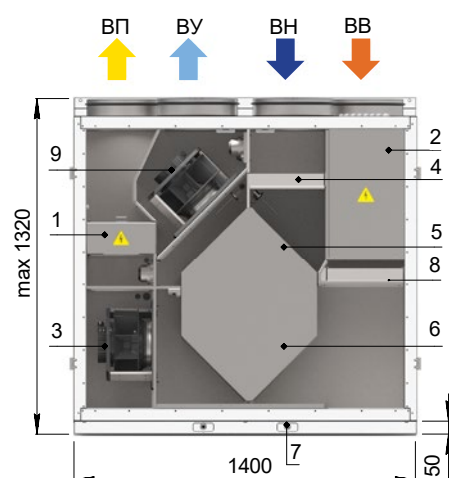
Вид F
