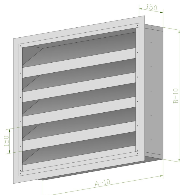
АКУСТИК 1-150 с/ф АхВ – размеры строительного проема
