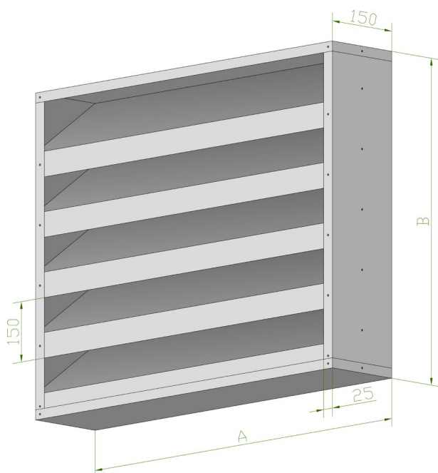
АКУСТИК 1-150 б/ф АхВ – габаритный размер решетки
