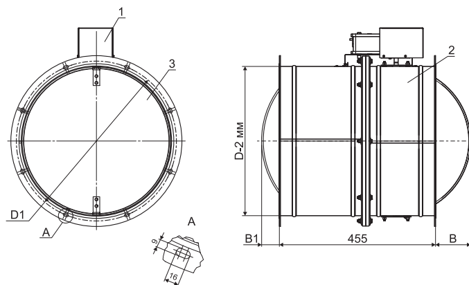
Клапан на фланце
