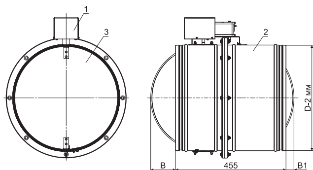
Клапан на ниппеле
