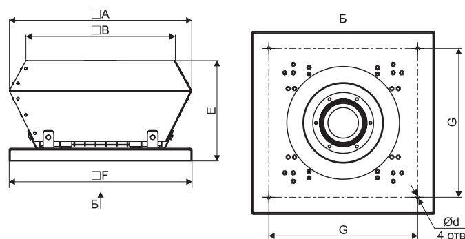
ВКРФ-М с колесом GH
