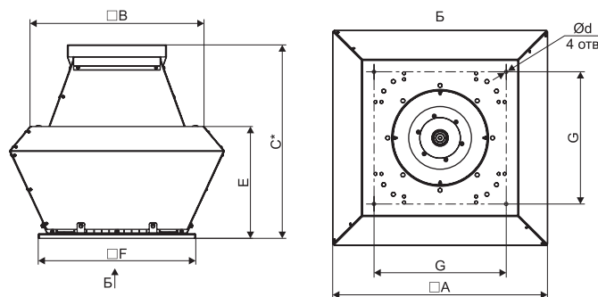
ВКРФ-М с колесами PH, PC
